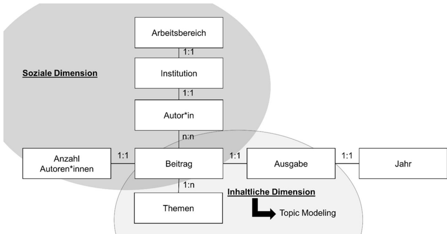
Abb. 3 Vereinfachte Datenstruktur
